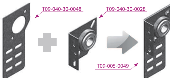
Sestava levé propojovací konzole
