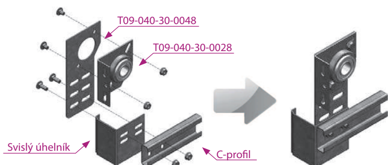
Uchycení propojovací konzole
